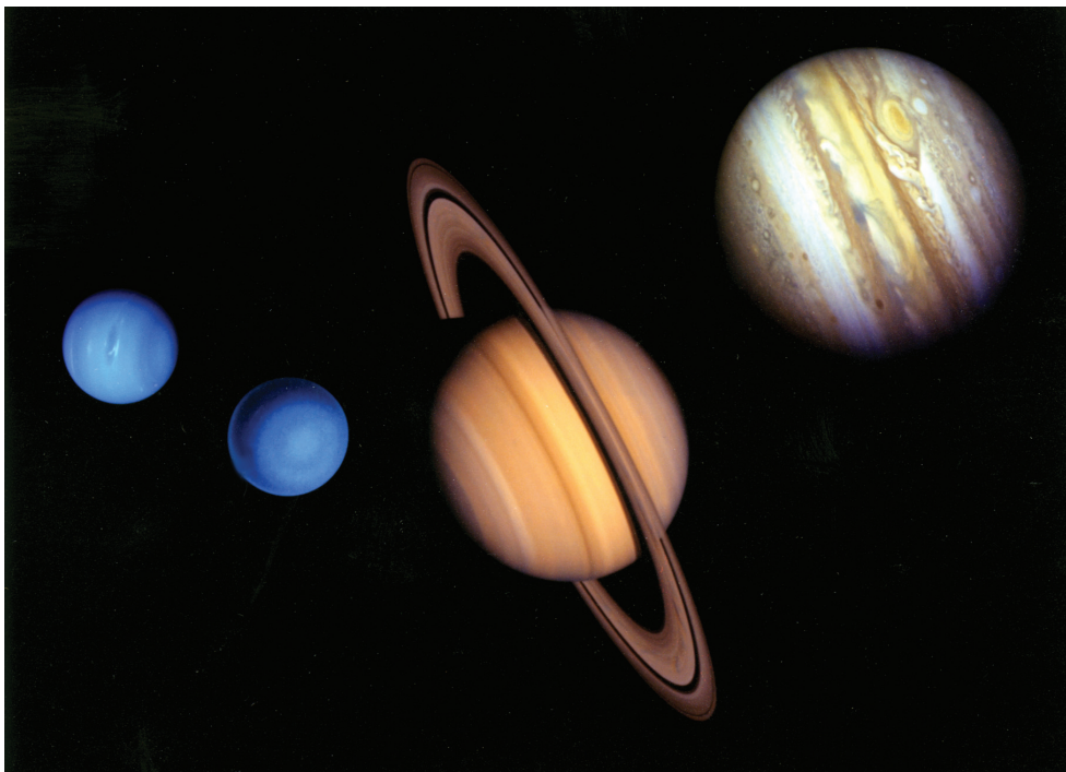
2- Montagem de imagens dos planetas gasosos, obtidas pela sonda espacial Voyager 2 nos anos de 1980. Da esquerda para a direita, vemos Netuno, Urano, Saturno e Júpiter (NASA/JPL).
