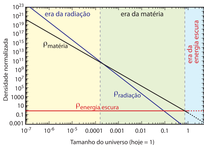
19- Evolução da densidade ( \rho ) das três principais componentes do Universo: energia escura, matéria (escura e bariônica), e radiação. As eras são definidas pela interseção da reta representando a densidade de matéria com a densidade de radiação e a densidade de energia escura.
