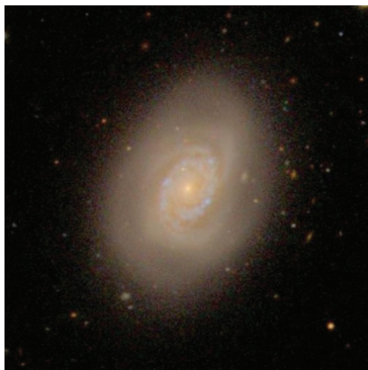
NGC 4580, espiral de tipo Sa
