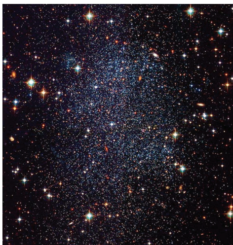
16- Esquerda: Imagem do telescópio Espacial Hubble da galáxia anã irregular de Sagitário (SagDIG), localizada a 3,5 milhões de anos-luz, descoberta em 1977. Direita: Galáxia anã de Cetus (constelação da Baleia), a 2,8 milhões de anos-luz, descoberta em 1999.
