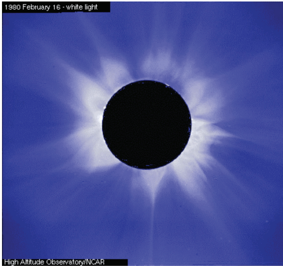
23- Elmos coronais, com suas formas pontiagudas ( http://umbra.nascom.nasa.gov/spartan/the_corona.html ).
