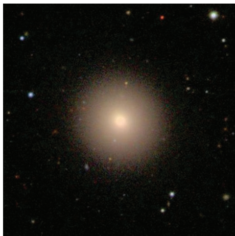
8- Galáxia E0, NGC 5198 (imagem do SDSS).
