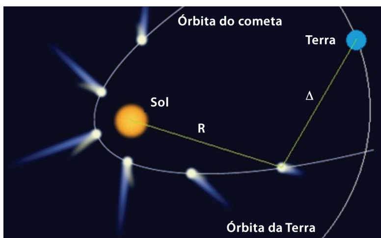
22- O brilho aparente de um cometa depende simultaneamente da sua distância ao Sol ( R ) e da distância dele à Terra ( D ).
