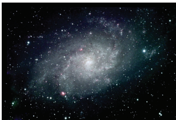
15- Esquerda: Galáxia de Andrômeda. Uma imagem da Lua foi colocada ao lado de M31 para dar uma ideia do seu tamanho aparente no céu. A olho nu, em uma noite muito favorável, pode-se observar a parte central do bojo como uma fraca nebulosidade no céu. Direita: galáxia do triângulo, M33.
