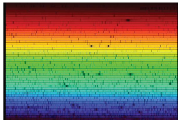
6- Espectro do Sol. A sequência de cores da azul ao vermelho representa a distribuição de cores da luz visível do Sol, divididas em cerca de 50 "fatias" horizontais, cada uma representando uma faixa de comprimentos de onda. As pequenas faixas escuras verticais são linhas ou bandas de absorção, cada uma delas provocada pela presença de um determinado íon ou molécula na superfície do Sol (crédito: Nigel Sharp – NOAO).
