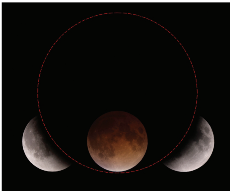
1- Sombra da Terra durante o eclipse lunar total de 09/11/2003 (Thierry Legault, http://legault.perso.sfr.fr/eclipse031109.html , data 21/02/2011).
