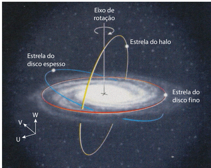
14- Órbitas das estrelas na Galáxia (C. Chiappini).
