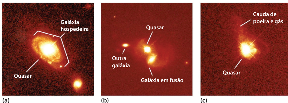
29- Imagens de quasares feitas com o telescópio espacial Hubble (HST), mostrando a galáxia hospedeira. Em vários casos constatou-se que a galáxia com um quasar interagia com uma vizinha. Apenas com imagens de ótima qualidade pode-se distinguir a galáxia de seu quasar, caso contrário o quasar literalmente ofusca a galáxia.
